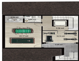
PLANTA SÓTANO
